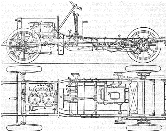
Остовъ автомобиля въ 24 лошадины силы: О—холодильникъ для воды; А—двигатель; В—механизмъ управленія; Е—выпускъ отработавшихъ газовъ; У—маховикъ, содержащій фрикціонную муфту; Р—педаль тормоза; Х—педаль разобщенія фрикціонной муфты; Т—педаль для увеличенія впуска газа въ двигатель; Л—ручной тормазъ; К—карбюраторъ; В—рессоръ, удерживающій фрикціонную муфту; Q—алюминіевый шпикъ, содержащій 4 пары шестеренъ для перемѣны передачъ и дифференціалъ; Q—тормазъ; S—глушитель, для уменьшенія шума выхода отработавшихъ газовъ; D, D—шестерни для пѣней ведущихъ колесъ.
